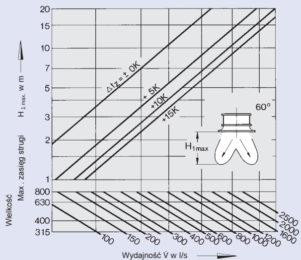
6 Maksymalny zasięg strugi przy nawiewie pod kątem 60°
