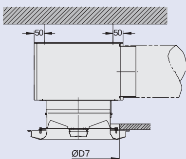
VDL-B-H (z kołnierzem)
