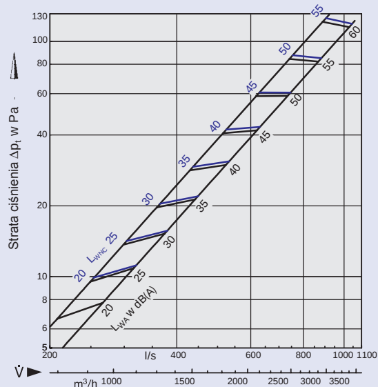
4 Poziom mocy akustycznej i strata ciśnienia Wielkość 800
