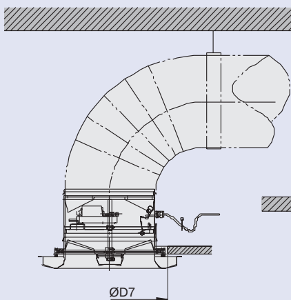
VDL-B-V (z kołnierzem)
