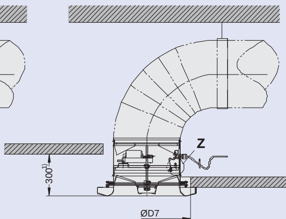
VDL-A-V (bez kołnierza)
