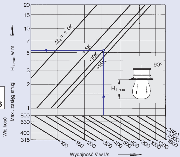
8 Maksymalny zasięg strugi przy nawiewie pionowym
