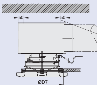
VDL-A-H (bez kołnierza)
