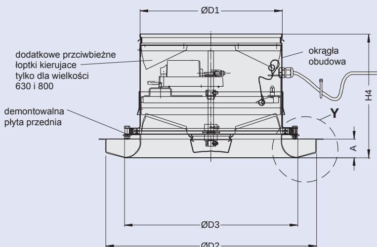
VDL-...-V (VDL-B-V-D-E1...E3 przekrój)
