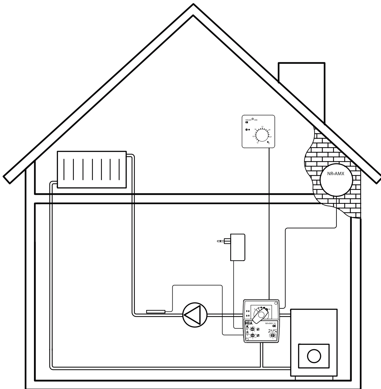
POMIESZCZENIOWY REGULATOR TEMPERATURY NR-AMX 10 RB
